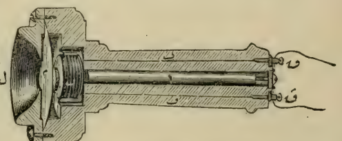
{ تلفون - ناقل صدا آخذه سی }
